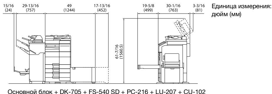
Основной блок + DK-705 + FS-540 SD + PC-216 + LU-207 + CU-102
