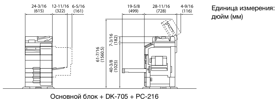
Основной блок + DK-705 + PC-216
