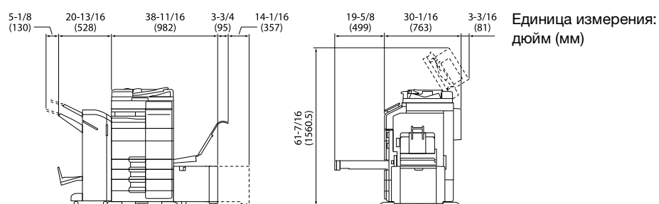
Основной блок + DK-705 + FS-539 SD + PC-216 + LU-302 + MK-730 + CU-102
