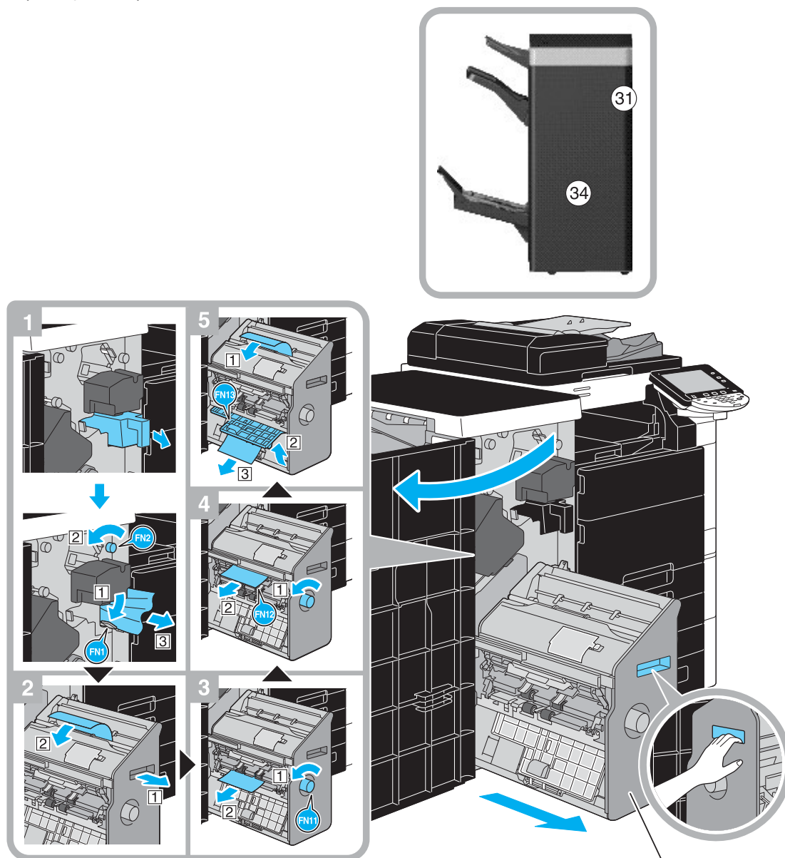
Устройство изготовления брошюр
