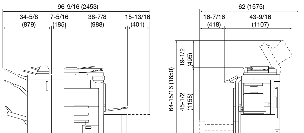
C652/C552 + FS-526 + SD-508 + ZU-606 + PI-505 + LU-301 Единица измерения: дюйм (мм)
