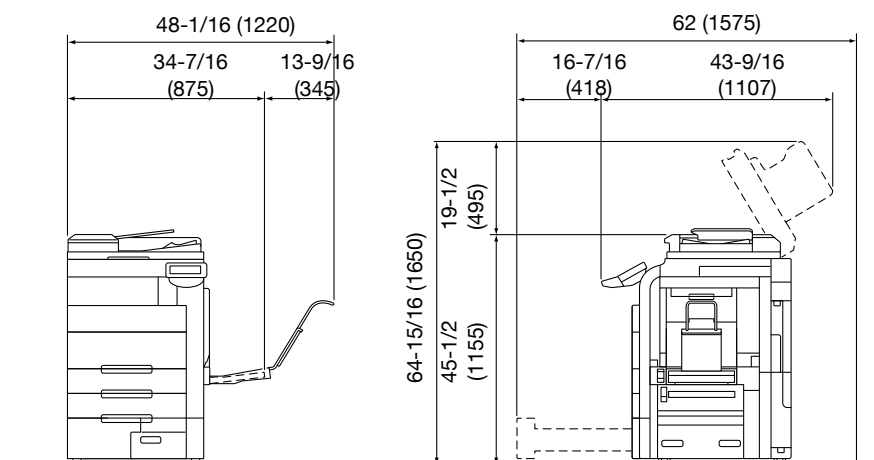
C652/C552 + MK-715 Единица измерения: дюйм (мм)
