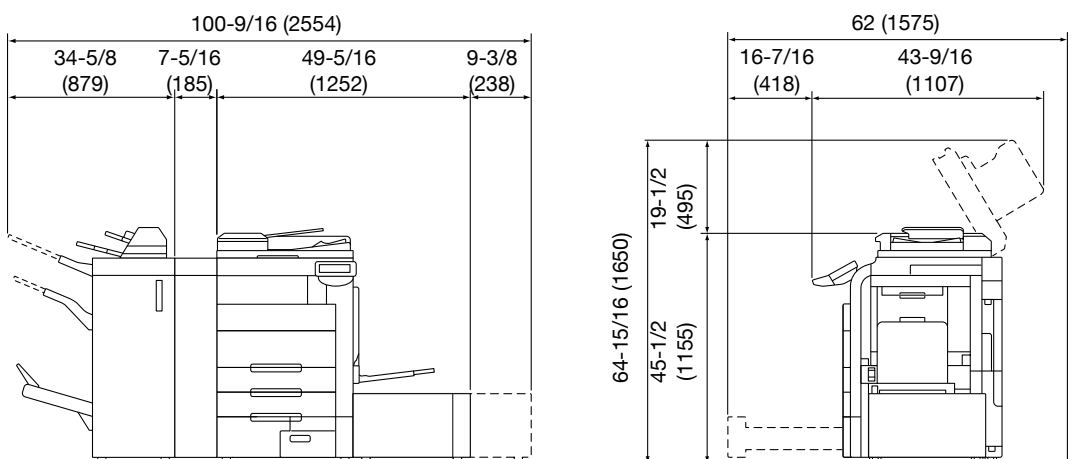
C652/C552 + FS-526 + SD-508 + ZU-606 + PI-505 + LU-204 Единица измерения: дюйм (мм)
