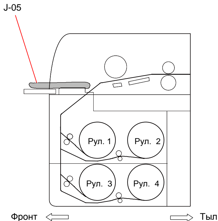
J-05 Стол ручной подачи
